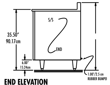
END ELEVATION
